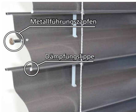
Lamellen werden wechselseitig durch vernietete Metallführungszapfen in den Schienen geführt Dämpfungslippe seitlich fixiert gegen Einziehen
