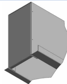
VUS - Vorbau-Unterputzschacht (Standard)
