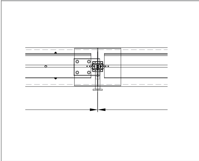
BSS - BLENDEN- UND SCHACHTSCHIEBESTOSS FÜR ALLE HÖHEN
