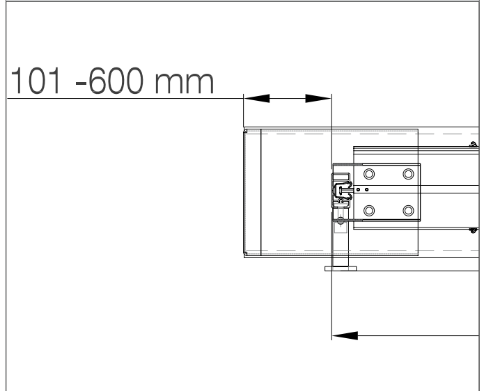
VLSAOS - EVOR VORSATZSCHACHT - LEERSCHACHT AUSSEN OHNE SEITENABSCHLUSS
