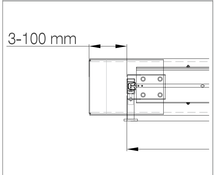
VSVMs - EVOR VORSATZSCHACHT - SCHACHTVERLÄNGERUNG MIT SEITENABSCHLUSS
