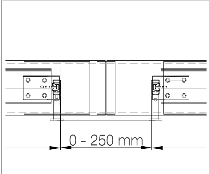
VSSSV - EVOR VORSATZSCHACHT - SCHIEBESTOSS MIT SCHACHTVERLÄNGERUNG
