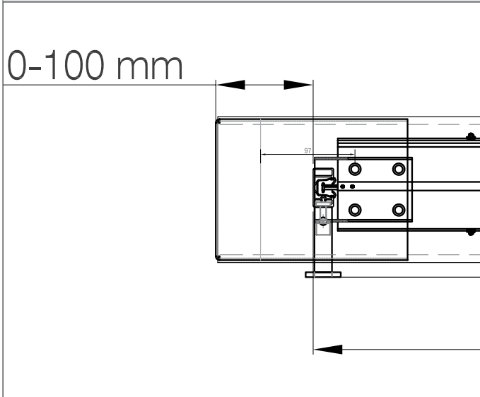
VSVOS - EVOR VORSATZSCHACHT - SCHACHTVERLÄNGERUNG OHNE SEITENABSCHLUSS
