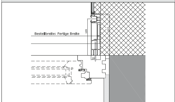
VERTIKALSCHNITT EKRA MIT AUSFÜHRUNG SCHACHT VUS
