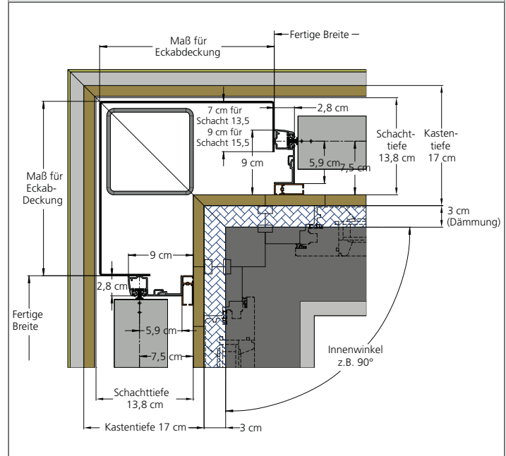
ISO-USI-28,5 | ISO-USI-33,5 | ISO-USI-41,5 14 cm SCHACHTTIEFE, ECKVERBLENDUNG
