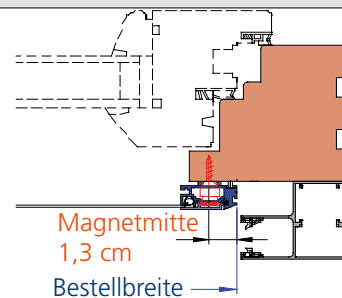
HORIZONTALSCHNITT IN VERBINDUNG MIT ROLLADEN DFSE
