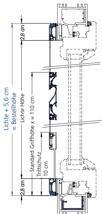
VERTIKALSCHNITT FÜR KUNSTSTOFFFENSTER
