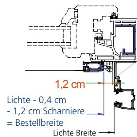
HORIZONTALSCHNITT SOFTFÜHRUNGSSCHIENE
