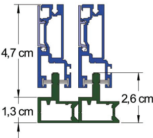
DETAIL BODENFÜHRUNG
