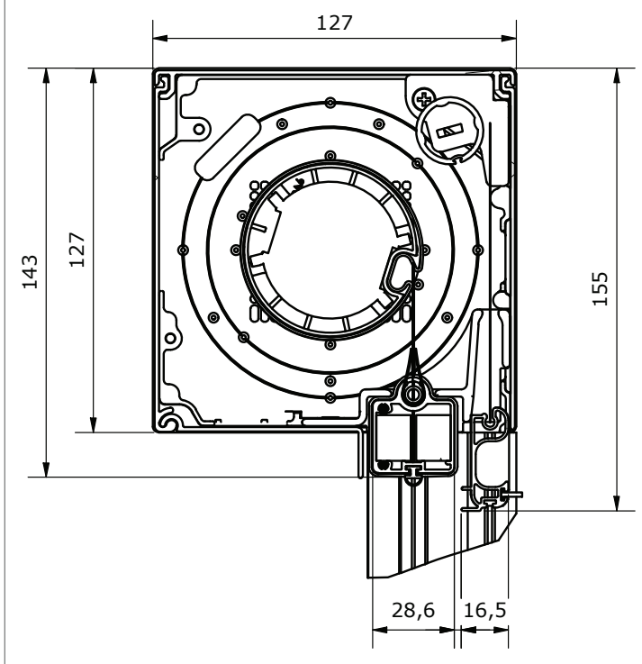
VERTIKALSCHNITT ZIP-AP MIT ZRCI-H-NF
