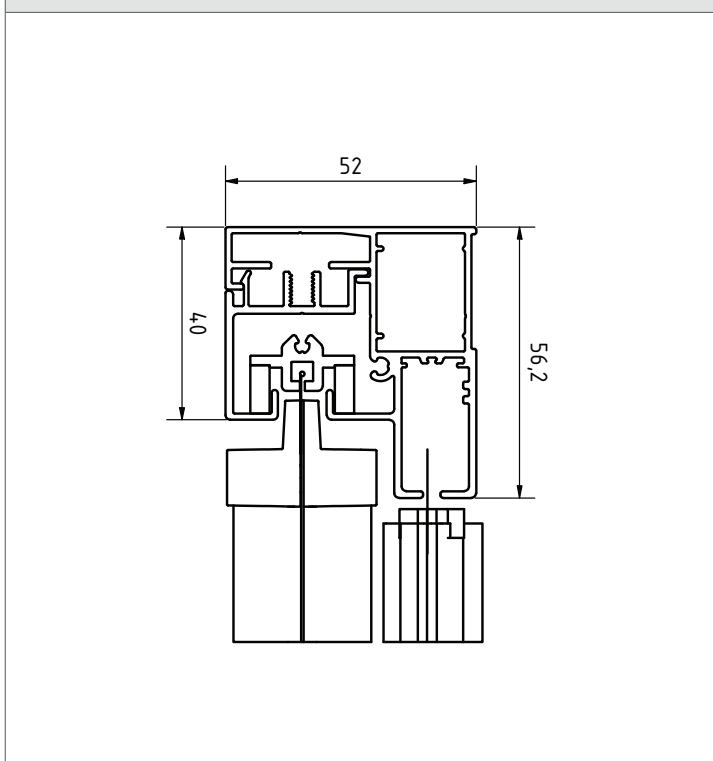
HORIZONTALSCHNITT ZIP-AP MIT ZRCI-H-NF
