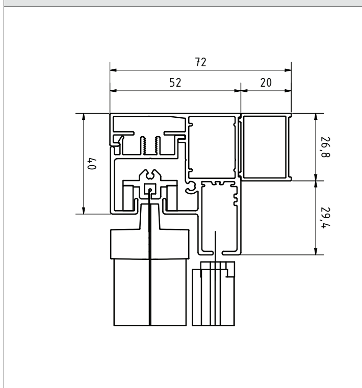
HORIZONTALSCHNITT ZIP-UP MIT ZRCI-H-NF
