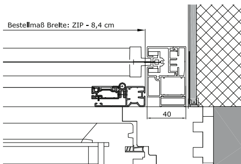
HORIZONTALSCHNITT ZIP-AP KOMBINATION ISS112 UND ISS113
