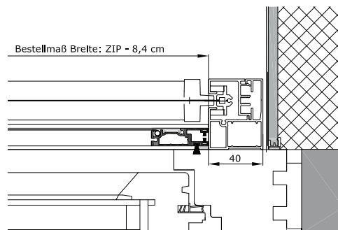
HORIZONTALSCHNITT ZIP-AP KOMBINATION SCHIEBERAHMEN ISS114
