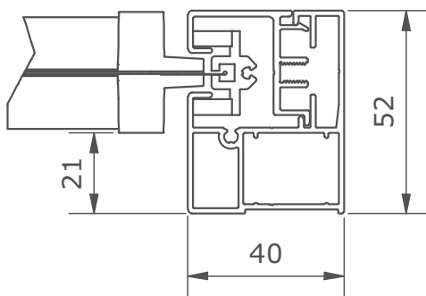
HORIZONTALSCHNITT FÜHRUNGSSCHIENE BEMESSUNG ENGLEISTE
