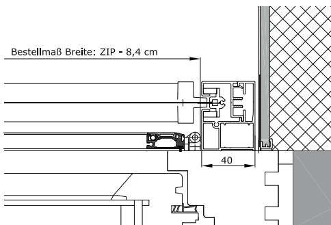
HORIZONTALSCHNITT ZIP-AP KOMBINATION SCHWENKRAHMEN ISS111
