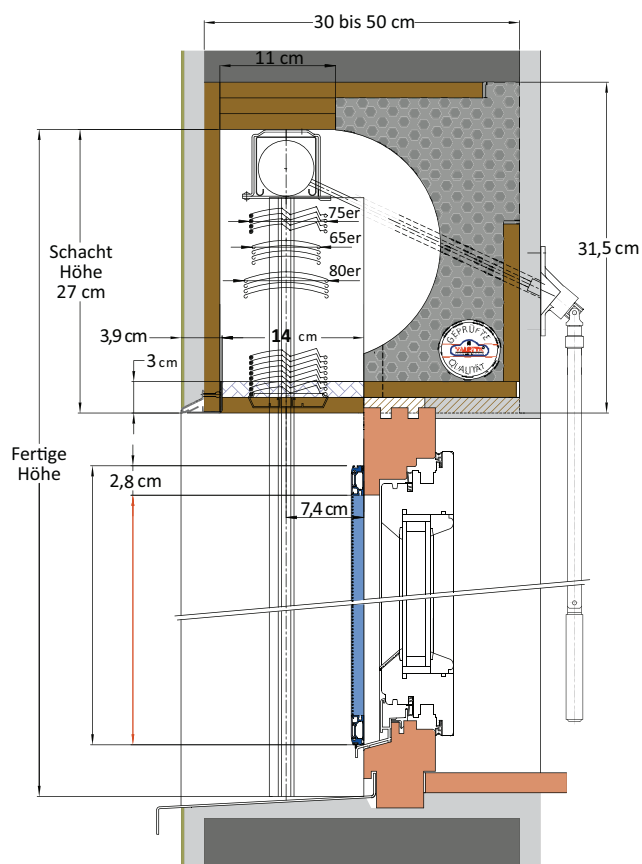
VERTIKALSCHNITT ISO-KRA IN KOMBINATION MIT ISS108 FÜR HOLZFENSTER MIT ALU- FENSTERBANK
