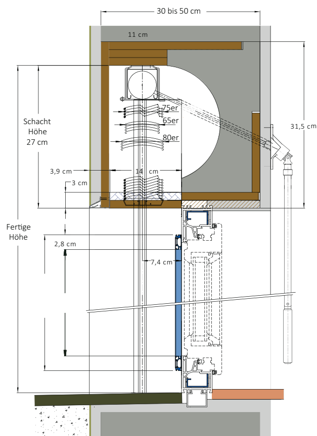
VERTIKALSCHNITT ISO-KRA IN KOMBINATION MIT ISS108 FÜR KUNSTSTOFFFENSTER MIT HOLZFENSTERBANK
