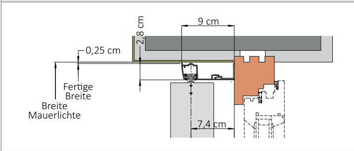
HORIZONTALSCHNITT ISO-KRA FÜR HOLZFENSTERSTOCK MIT ALU-FENSTERBANKANSCHLUSS
