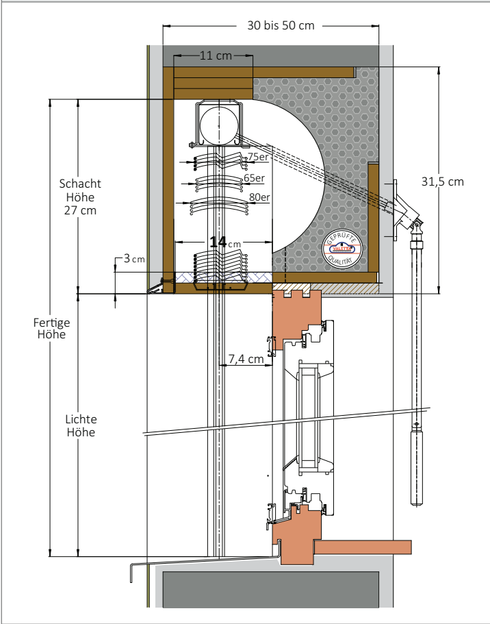
VERTIKALSCHNITT ISO-KRA FÜR HOLZFENSTER MIT ALUFENSTERBANK
