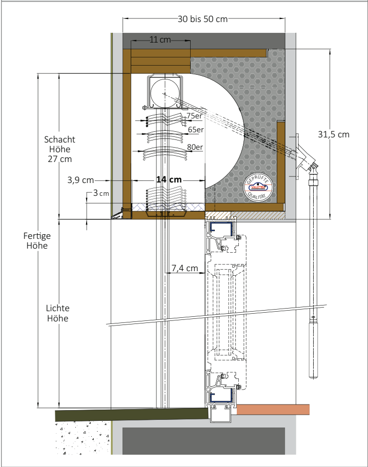
VERTIKALSCHNITT ISO-KRA FÜR KUNSTSTOFFFENSTER MIT HOLZFENSTERBANK
