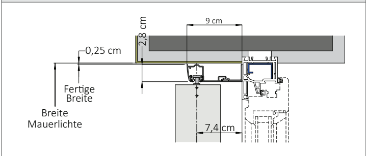
HORIZONTALSCHNITT ISO-KRA FÜR KUNSTSTOFFFENSTER MIT HOLZFENSTERBANK
