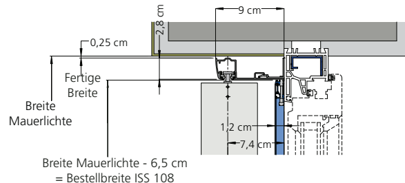
HORIZONTALSCHNITT ISO-KRA IN KOMBINATION MIT ISS108 FÜR KUNSTSTOFFFENSTER MIT HOLZFENSTERBANK
