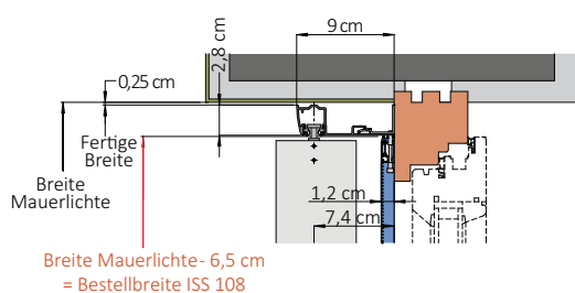
HORIZONTALSCHNITT ISO-KRA IN KOMBINATION MIT ISS108 FÜR HOLZFENSTER MIT ALU- FENSTERBANK
