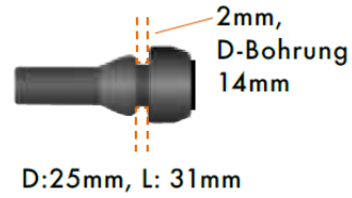
Abb. 3. Schutzülle für Netzgeräte-Anschlussbuchse, die Buchse wird darin eingedrückt und diese kann dann hiermit versenkt montiert werden, um eine Nachladung leicht von außen, bei geschlossenem Kasten vornehmen zu können, mit Abdeckkappe.
