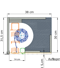
ISO ROLLRAFF NEUBAUSTURZKASTEN
