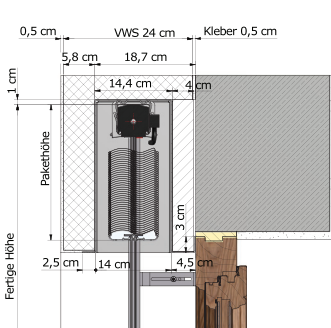
VUS-VORBAU UNTERPUTZSCHACHT
