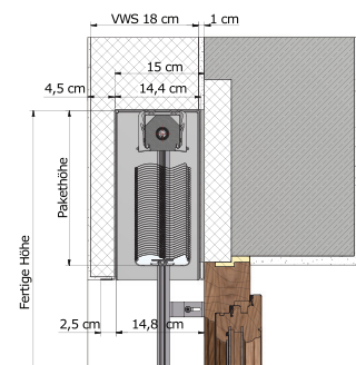
AUS-AUFSATZ UNTERPUTZSCHACHT
