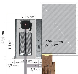
ISO-EPS-PLUS VORBAUELEMENT
